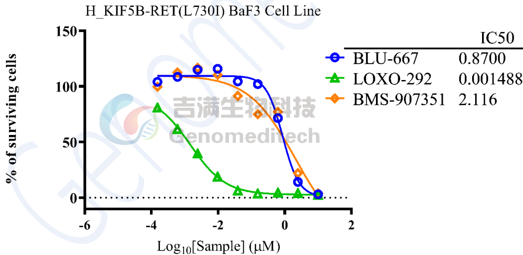
Fig 1. H_KIF5B-RET(L730I) BaF3 Cell Line 使用 BLU-667、LOXO-292 、BMS-907351 杀伤验证结果。换算方法: 活细胞百分比= (加药孔-assay buffer 孔) / (不加药孔-assay buffer 孔)
